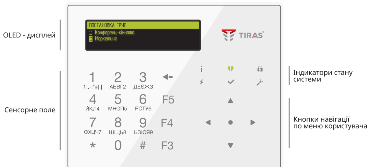
Рисунок 2.1 – Клавіатура K-GLCD
