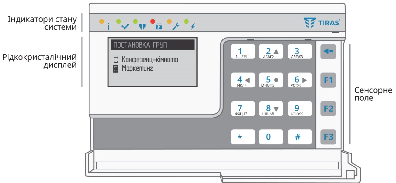
Рисунок 2.2 – Клавіатура K-LCD
