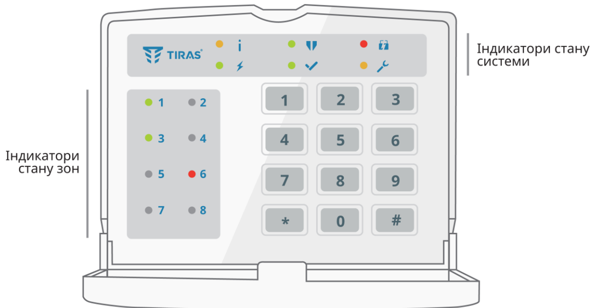
Рисунок 2.3 – Клавіатура K-LED8
